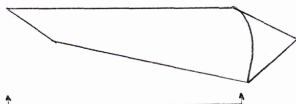
Rayons lumineux
